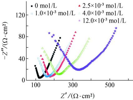
(b) 带锈铸铁
