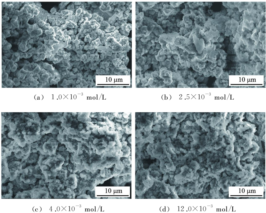
图 9 不同浓度儿茶素处理后铸铁表面锈层的扫描电镜图
