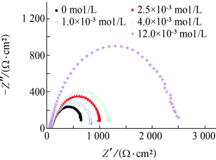
(a) 裸铸铁
