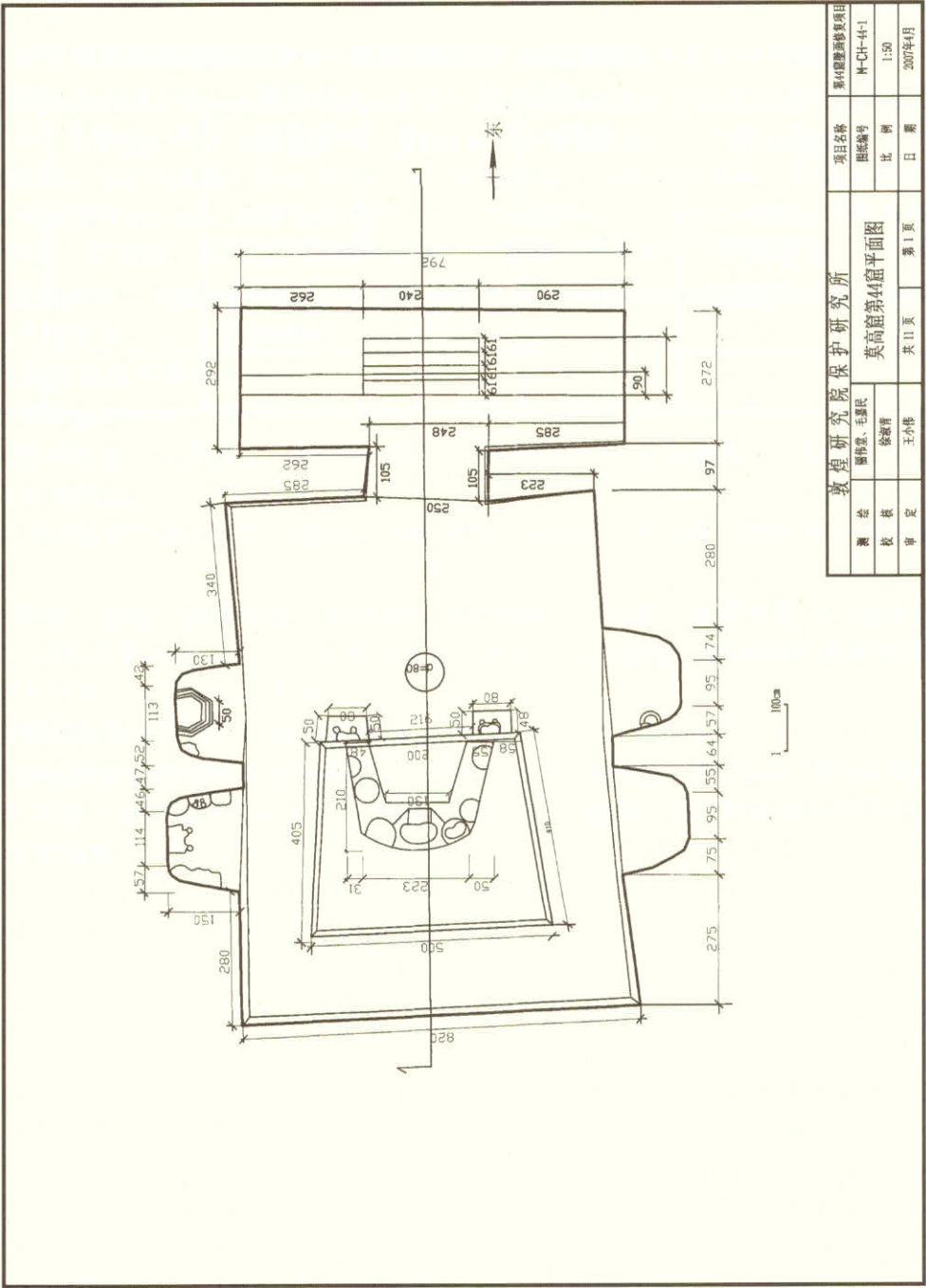
图 B.1 洞窟平面测绘示例图
